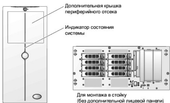
Рисунок 1-1. Корпуса системы: для монтажа в стойку и в виде вертикального блока
